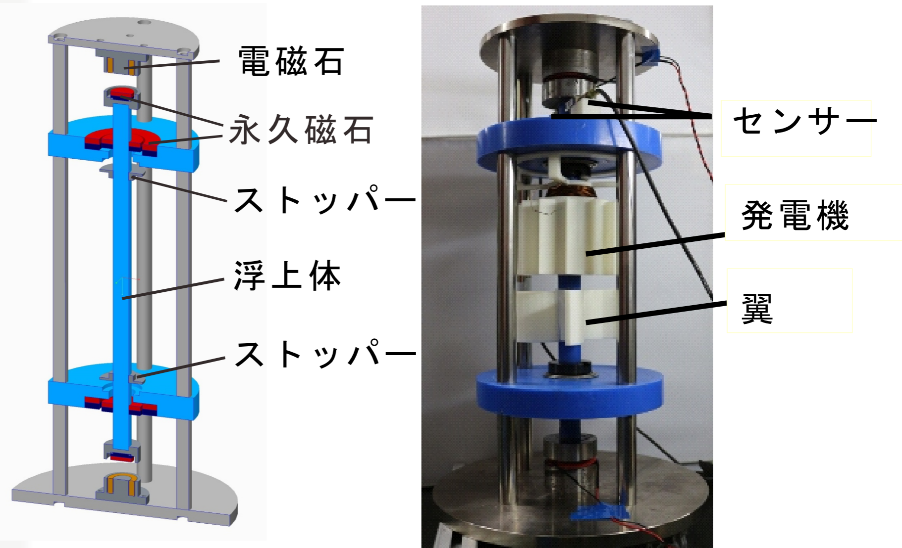
磁気浮上を利用した風力発電装置
